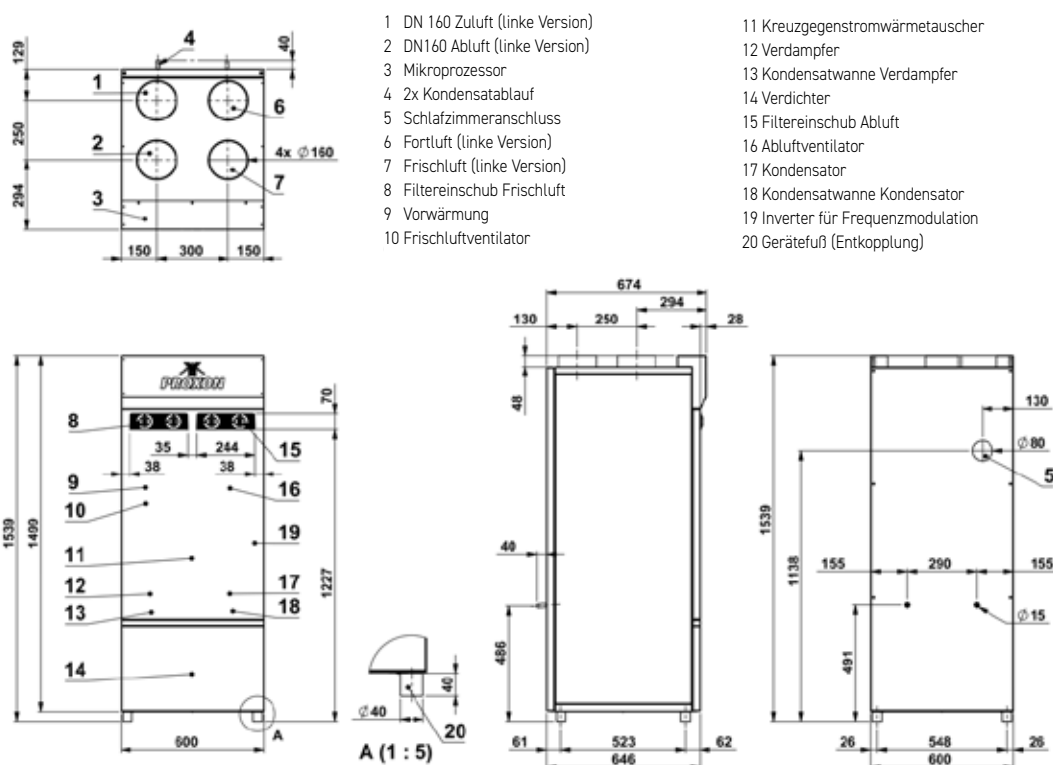
Abbildung: Variante „links“ Hinweis: Bei der rechten Version ändern sich folgende Anschlüsse: 1= Fortluft, 2= Frischluft. 6= Zuluft, 7= Abluft
