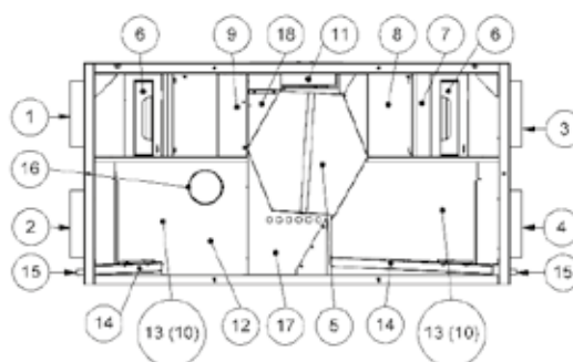
Ansicht von Vorne ohne Frontplatte
